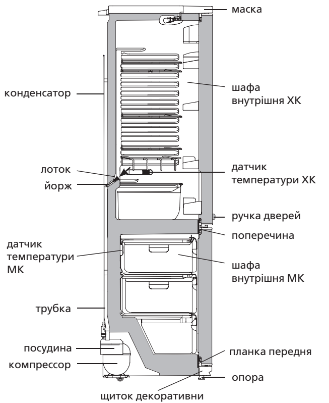
Рисунок 7 — Схема зливу талої води із ХК
